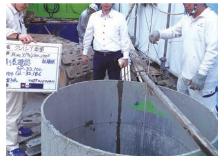
杭検査 支持層確認状況
