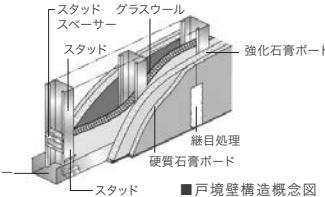
■戸境壁構造概念図
