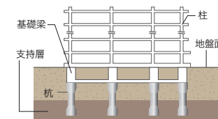
■杭基礎概念図
